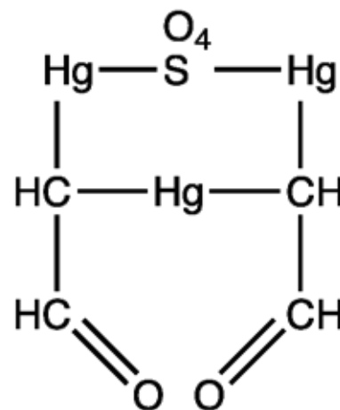
Figura 32. Catalizador que se forma en la reacción de hidratación del acetileno
