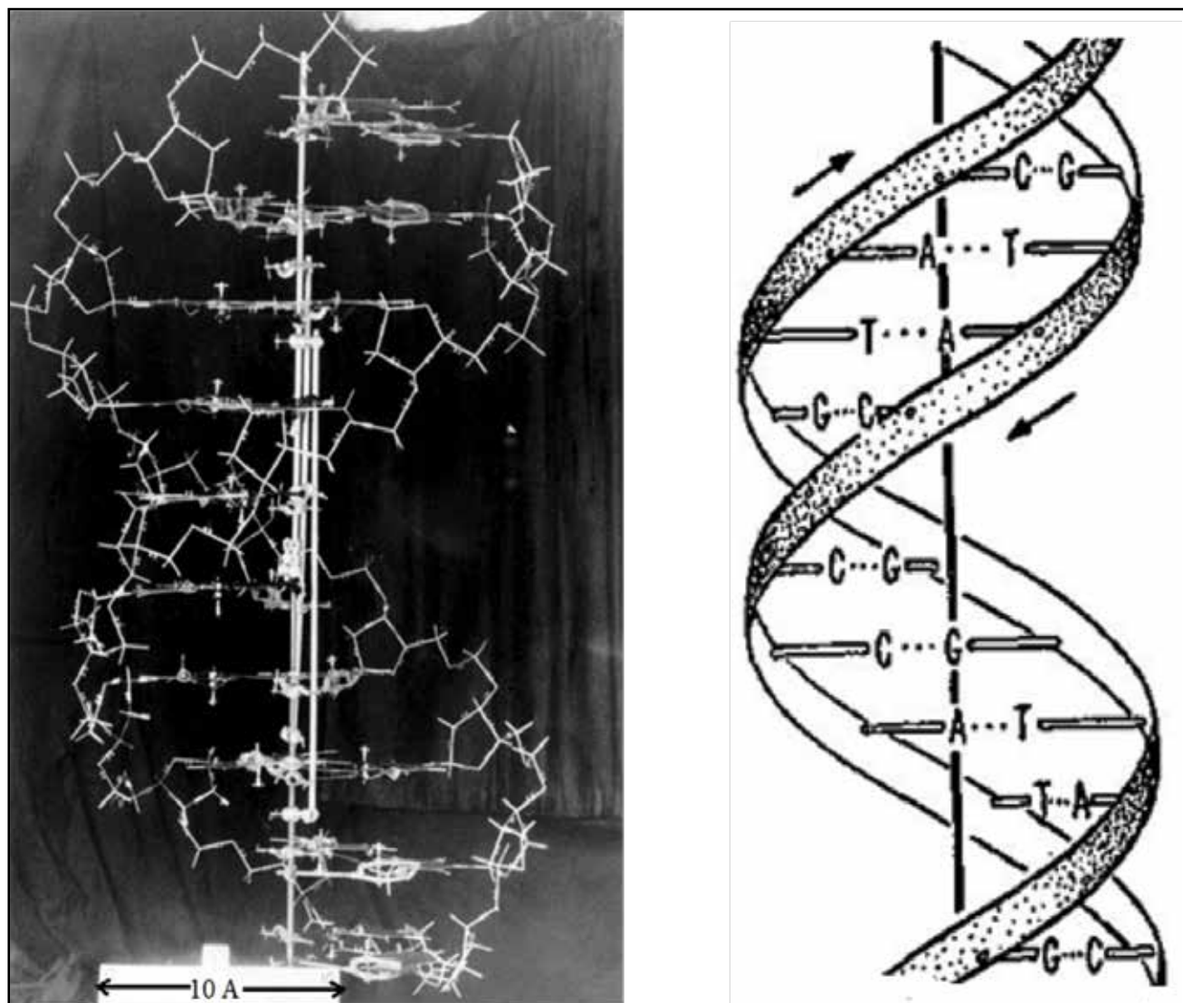
Figura 30: Izquierda: Modelo original en escala de Watson y Crick de la molécula de ADN-B (hecho de alambres y chapas). La tira horizontal al pie del modelo indica la magnificación del mismo y corresponde a una longitud de 10 Å. El modelo se extiende verticalmente un paso de la hélice (unos 34 Å). Derecha: esquema original del ADN (adaptado de Watson & Crick, 1953).
