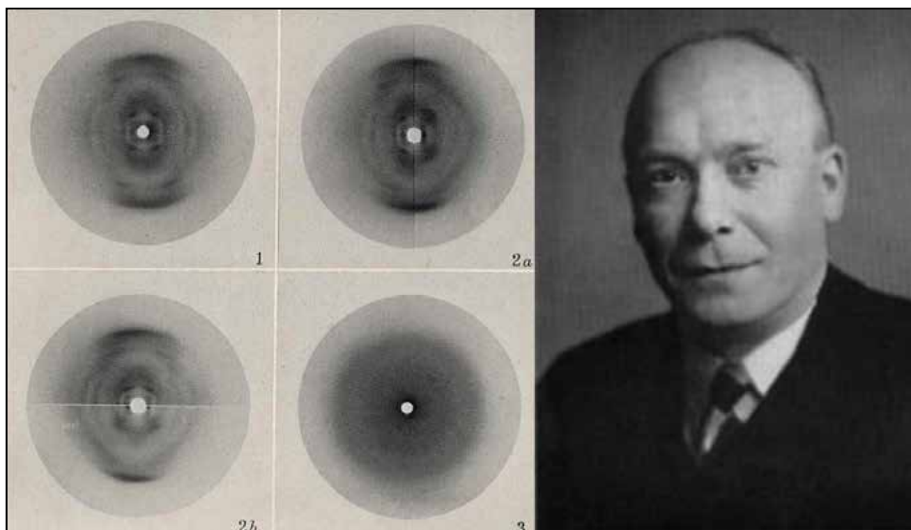
Figura 13: Izquierda. Placa 1: difracción de rayos-X en fibras (orientadas verticalmente) de la sal sódica de ADN extraído de timo de cabra (NaADN). Placas 2a,b: comparaciones de los patrones de difracción de ADN de cabra con ADN de arenque. El haz incidente es perpendicular a las fibras y al plano de las placas. Placa 3: difracción en polvos de ADN de levadura. Derecha: William Thomas Astbury (1898-1961).
