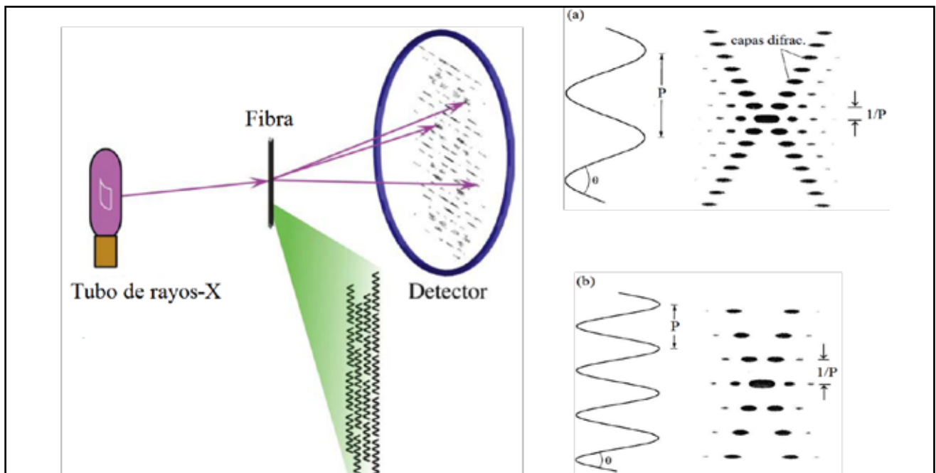
Figura 24: Izquierda: arreglo experimental para difracción de rayos-X en fibras de DNA-B. Derecha: relación recíproca entre el paso de hélices y sus correspondientes patrones de difracción.
