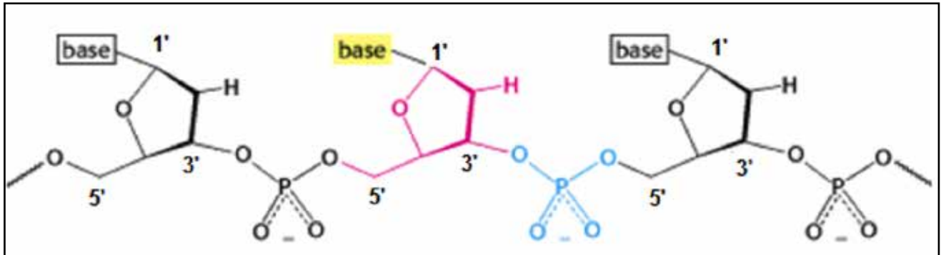
Figura 7: Estructura química de un poli-nucleótido de ADN.
