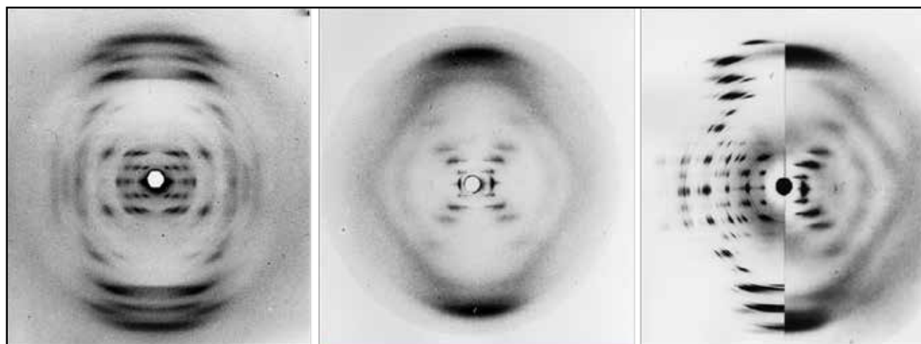
Figura 17: Izquierda: foto de difracción de rayos-X de ADN-A (75% humedad). Centro: foto de ADN-B (92% humedad). Derecha: comparación de ambos patrones.
