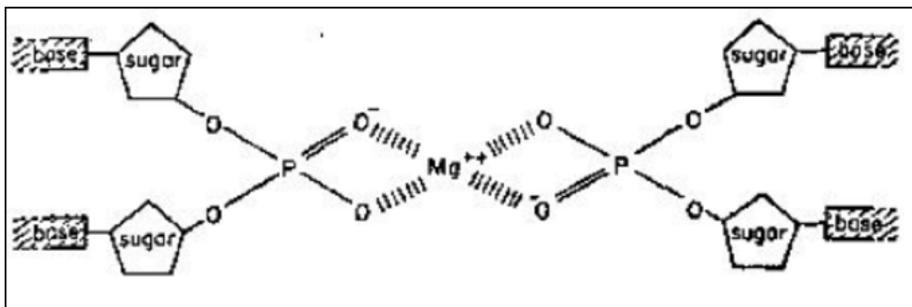
Figura 19: Esquema del modelo preliminar de ADN de Watson y Crick consistente en tres hélices (se muestran sólo dos) con las bases proyectándose hacia fuera y los grupos fosfatos hacia el eje helicoidal. La repulsión electrostática entre las cargas negativas de fosfatos próximos se vería compensada por iones Mg^{2+} coordinados.
