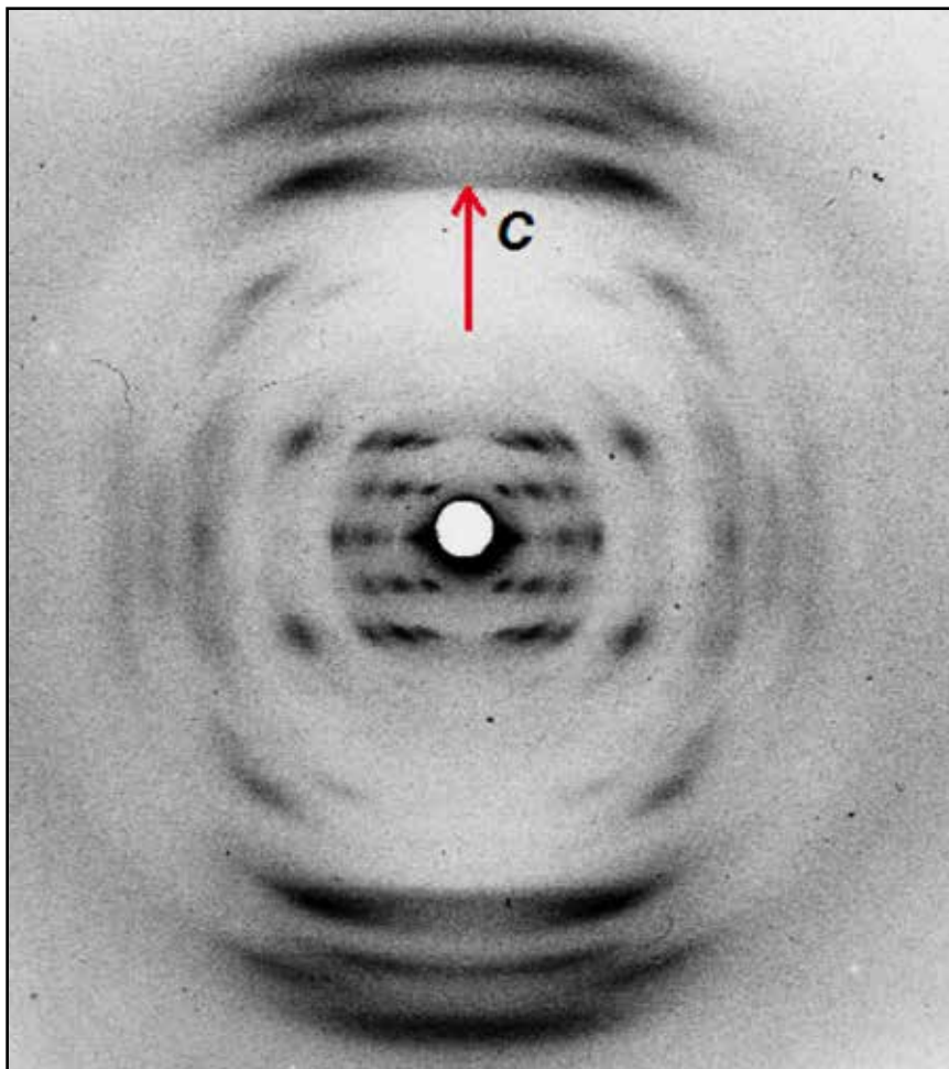
Figura 18: Fotografía de difracción de rayos-X de tres fibras (18-30 \mu\text{m} de espesor) de NaADN deshidratado (humedad relativa del 75%) mostrando la forma cristalina A del ácido nucleico. La foto fue tomada por Franklin y Gosling luego de una larga exposición (116 h).
