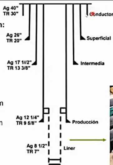
Figura 7: Características de la terminación de un pozo geotérmico (Massaro, 2020).
