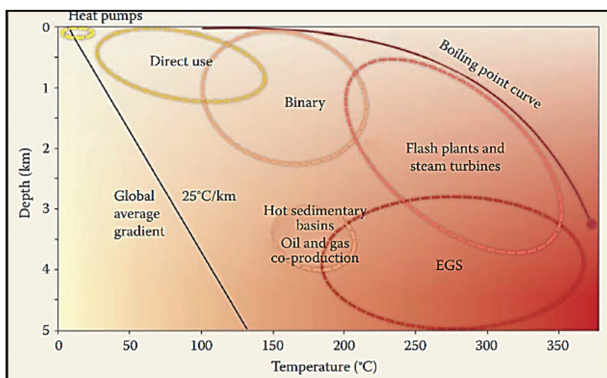
Figura 3: Gráfico de temperatura versus profundidad que muestra las distintas formas de aprovechamiento de la energía geotérmica, desde bombas de calor cercanas a la superficie terrestre hasta sistemas geotérmicos mejorados (Enhanced Geothermal Systems, EGS) que se encuentran en etapa temprana de desarrollo y se alcanzan a profundidades mayores a la de los reservorios generadores de energía que actualmente se están utilizando (Boden, 2017).
