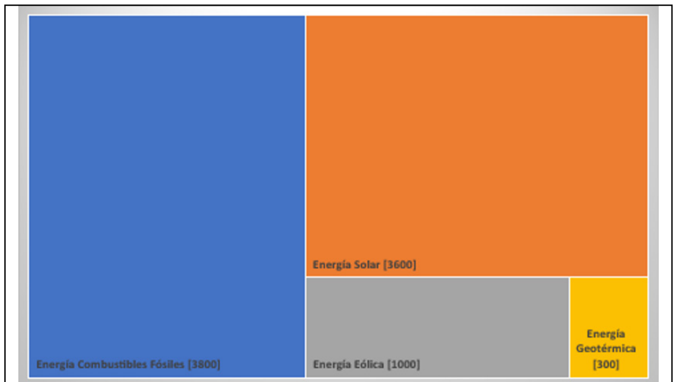
Figura 4: Uso de suelo de la generación de energía a partir de combustibles fósiles, sol y viento. Las unidades de los valores entre corchetes son m^2/MWh (Barcelona, 2020).
